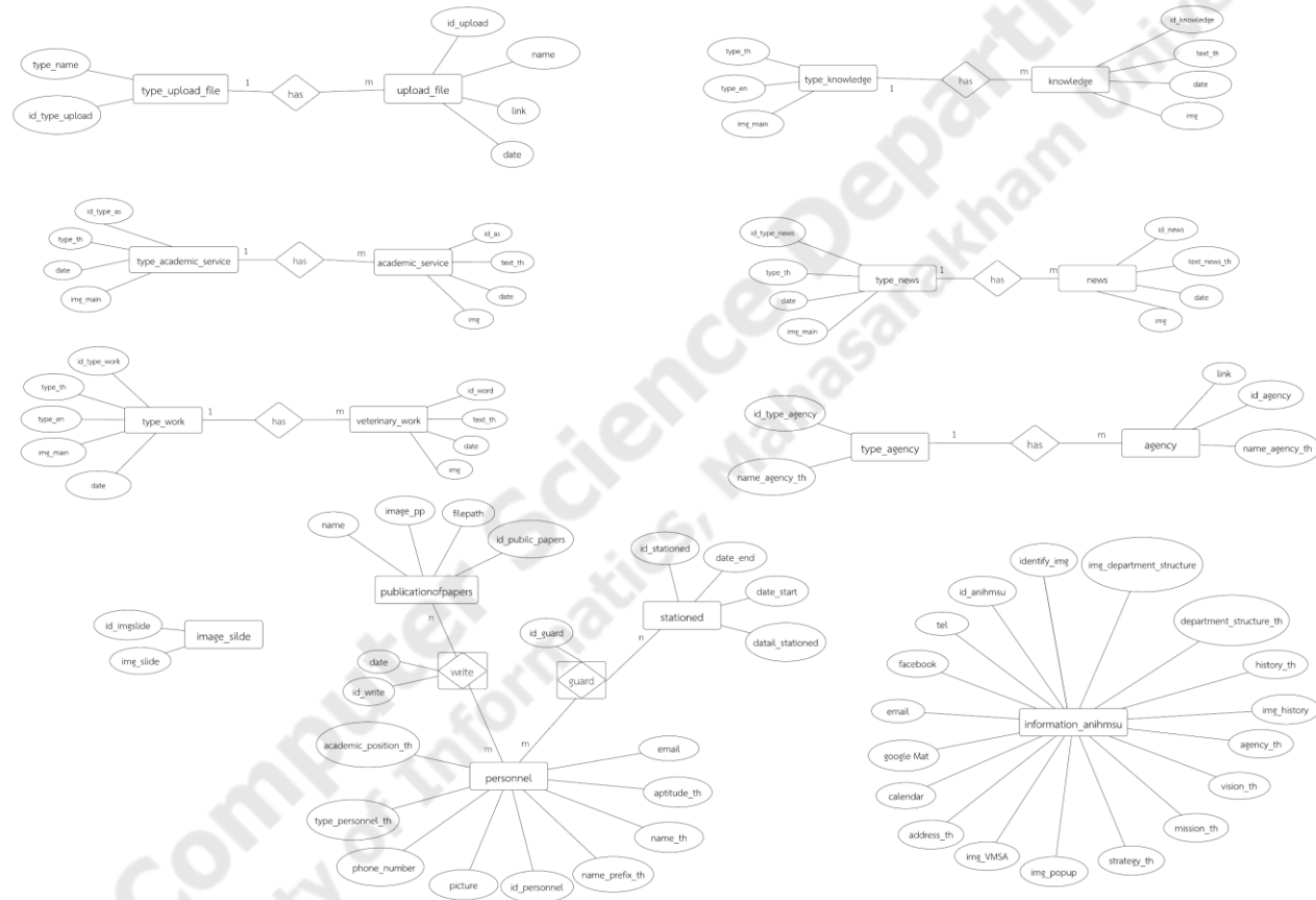
ภาพประกอบที่ 3.5 แผนภาพความสัมพันธ์ (Entities Relationship Diagram)
