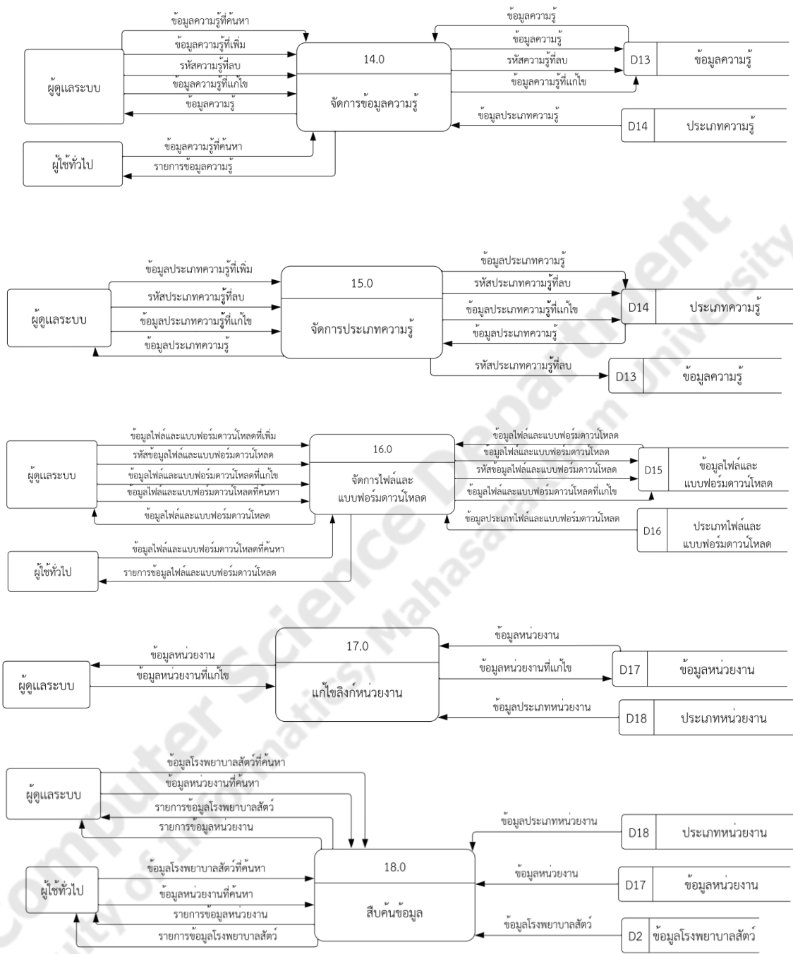
ภาพประกอบที่ 3.3 DFD level 1 (ต่อ)
