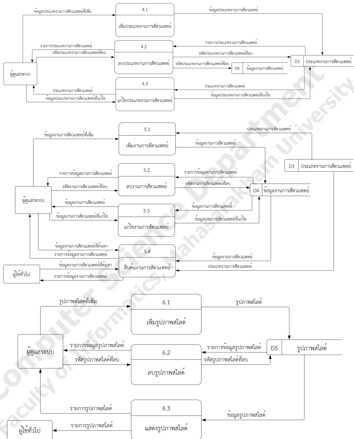
ภาพประกอบที่ 3.4 DFD level 2
