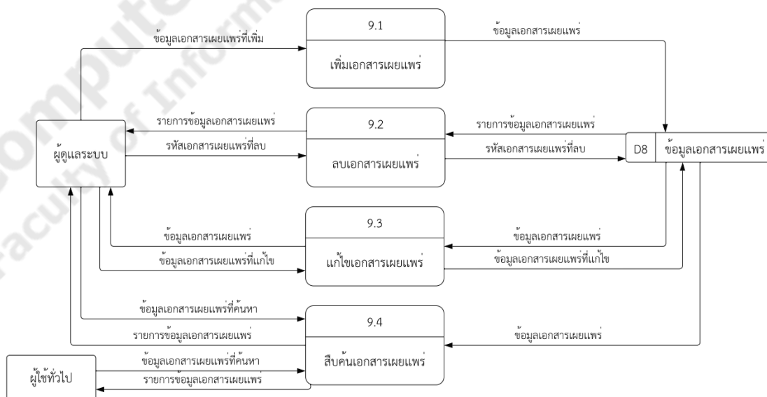
ภาพประกอบที่ 3.4 DFD level 2 (ต่อ)
