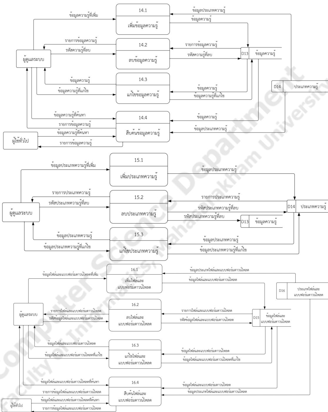
ภาพประกอบที่ 3.4 DFD level 2 (ต่อ)
