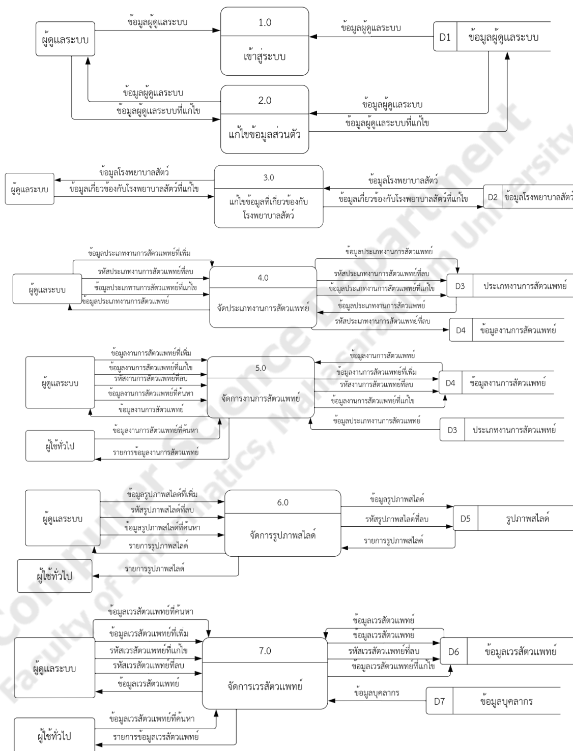
ภาพประกอบที่ 3.3 DFD level 1
