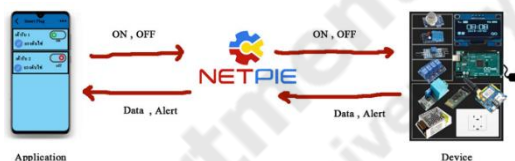
รูปที่ 4 การสื่อสารข้อมูลระหว่าง Smart Breaker และ MQTT (NETPIE)
